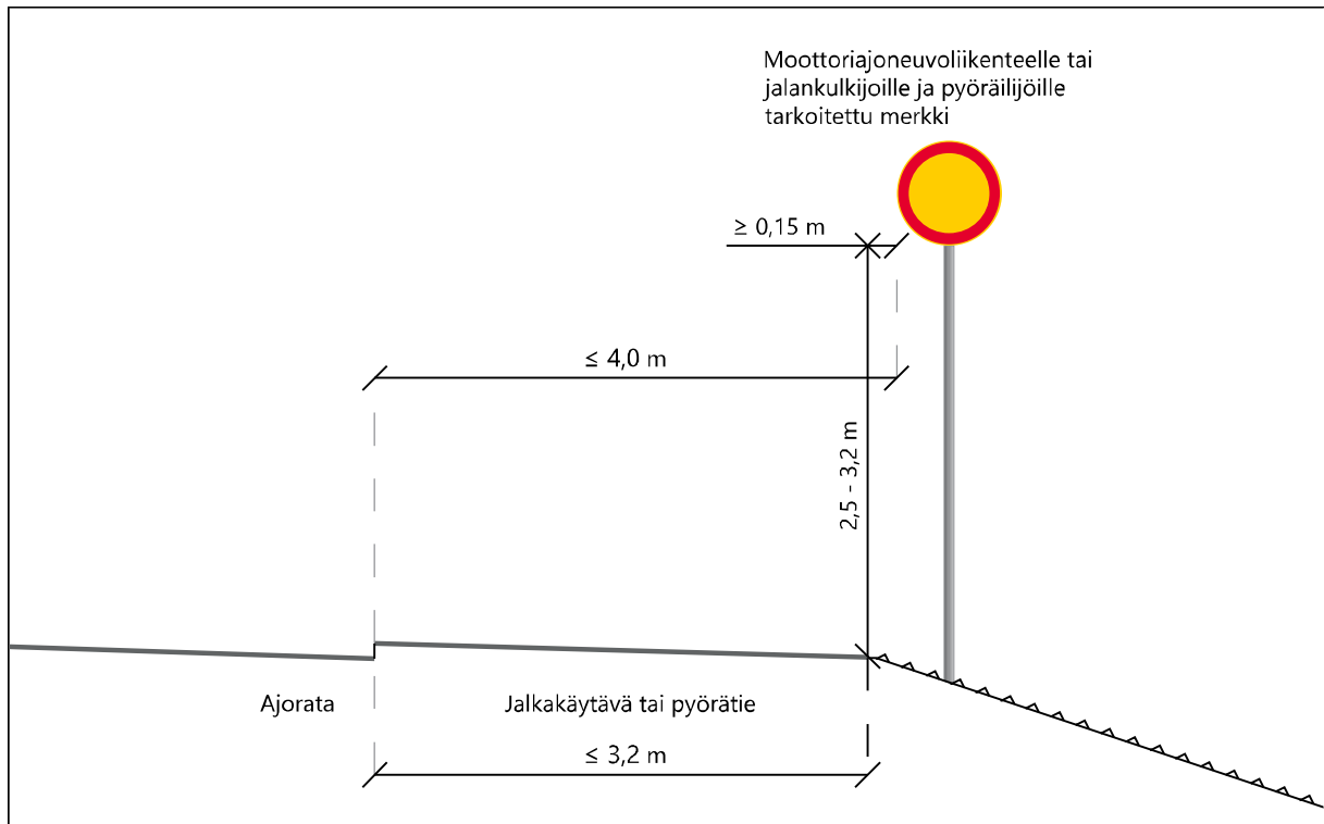
Kuva 1g. Liikennemerkkin sijoittaminen tien poikkileikkaukseen, kun tiehen liittyy enintään 3,2 metrin levyinen korotettu pyörätie ja jalkakäytävä, joka ei rajoitu sivuesteeseen.
