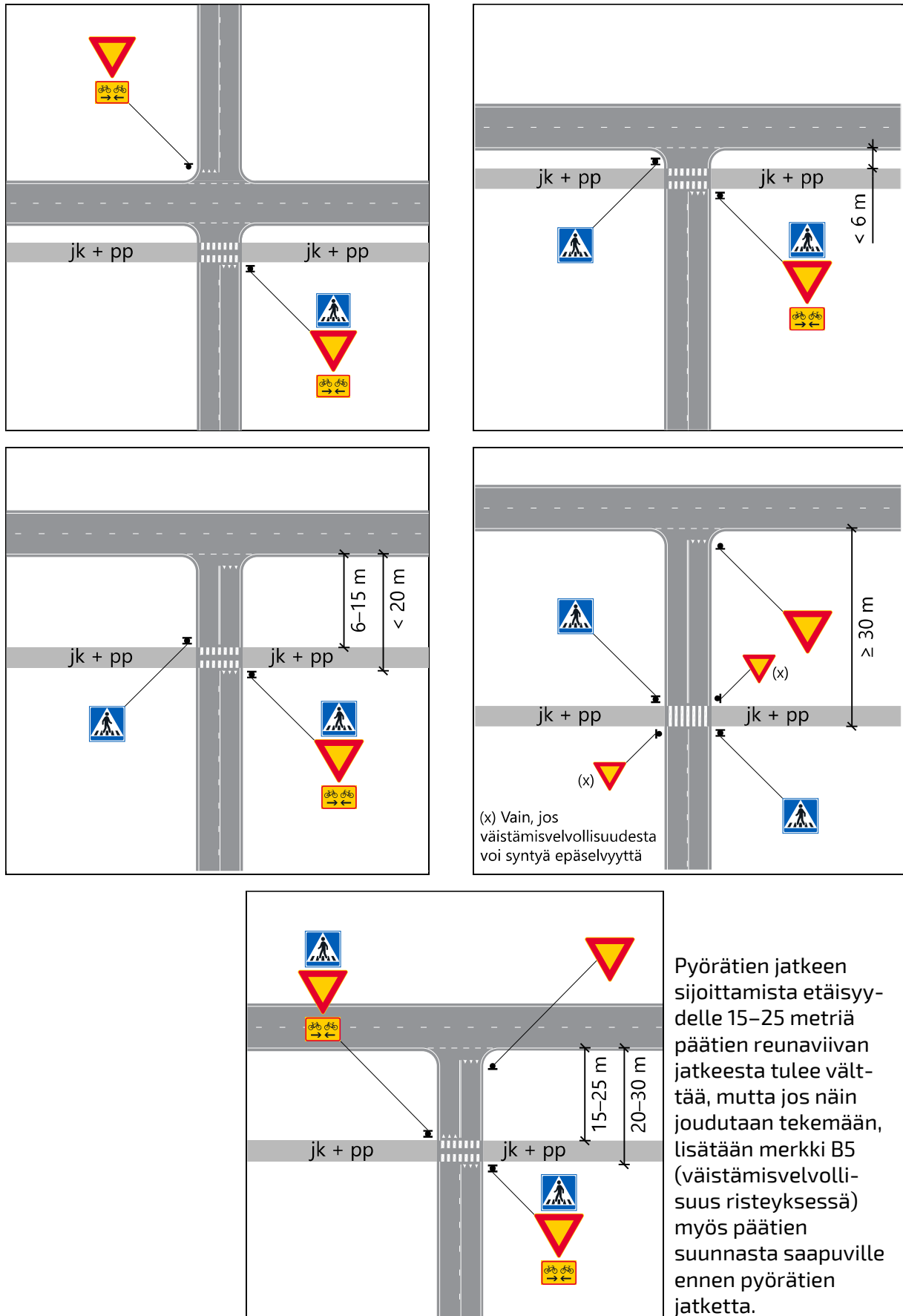
Kuva 33. Merkin B5 ja muiden liikenteenohjauslaitteiden käyttöperiaatteet pyörätien jatkeen sijaitessa eri etäisyyksillä päätien reunaviivan jatkeesta.
