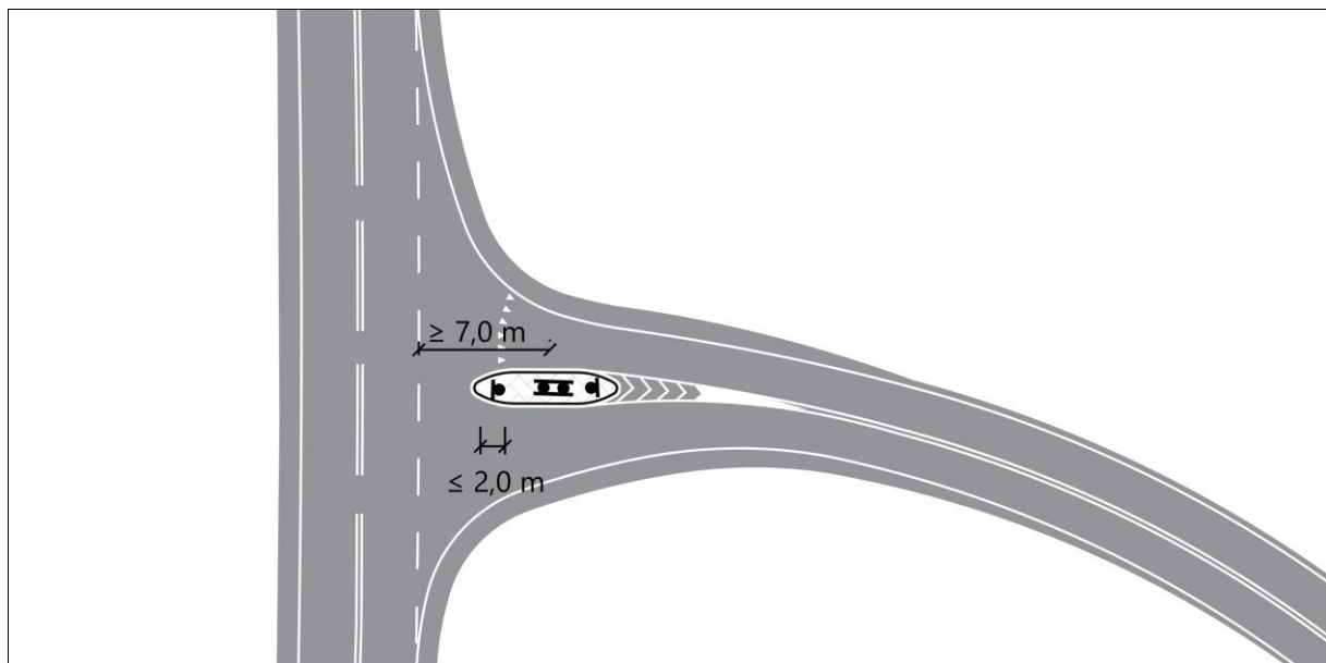
Kuva 4a. Tienviitan sijoittaminen liikenteenjakaajasaarekkeeseen. Viitta pyritään sijoittamaan korkeussuunnassa henkilöauton kuljettajan silmäpisteen yläpuolelle (viitan alareunan korkeus tien pinnasta yleensä vähintään 2,0 metriä).
