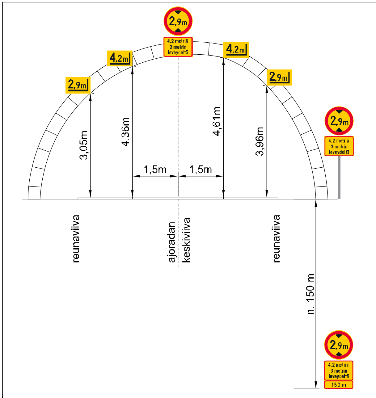
Kuva 166. Matalan holviaukon merkitseminen.
