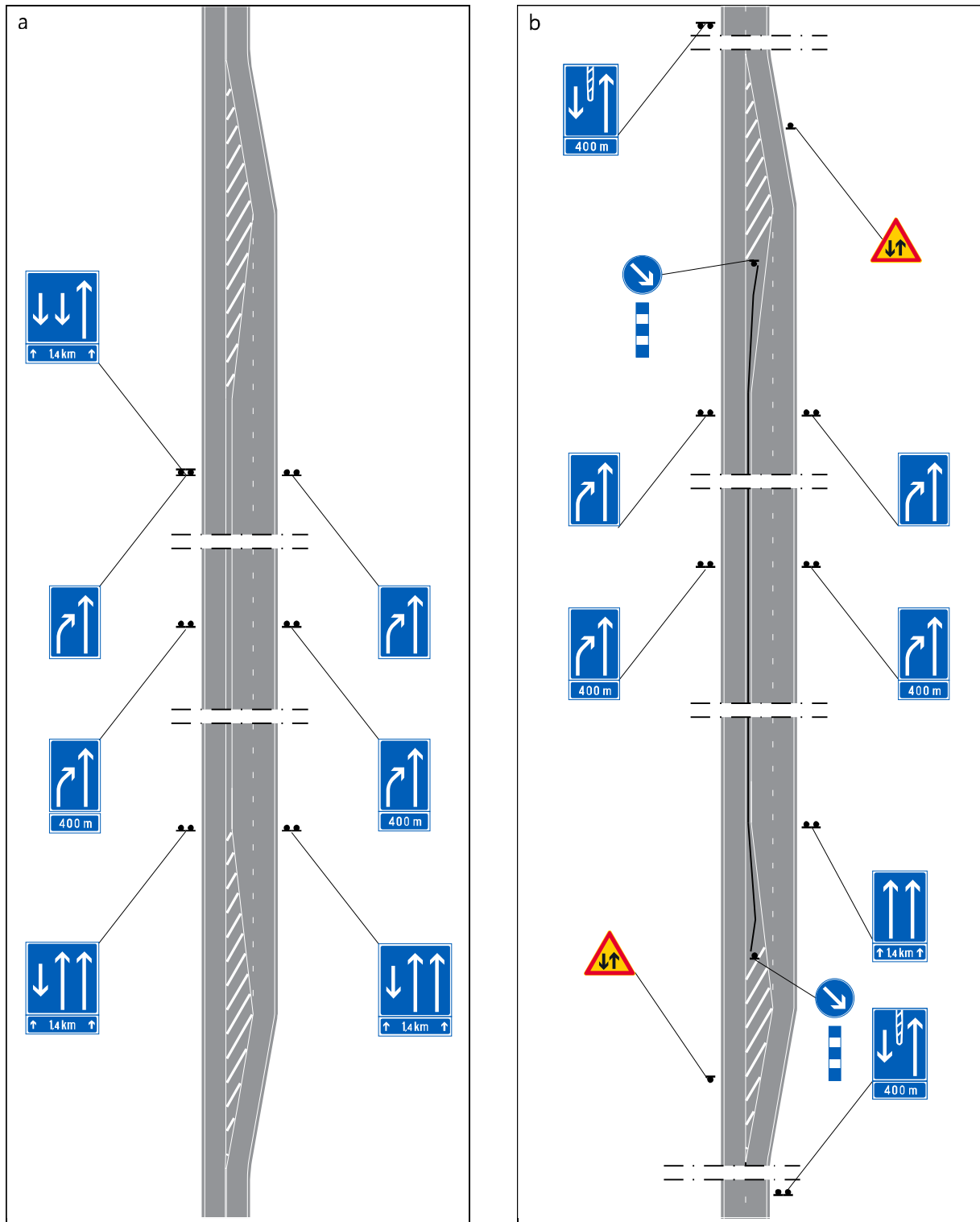
Kuva 119. 2+1 -ajokaistaisen ohituskaistan merkintäperiaate. Kuvassa a ajosuuntien välissä on kaksoissulkuviiva ja kuvassa b ajosuuntien välissä on kaide.
