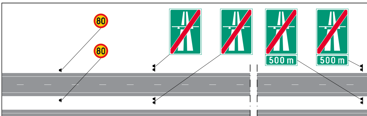
Kuva 99. Moottoritien päätymisen jälkeen tiekohtainen nopeusrajoitus osoitetaan merkillä C32.
