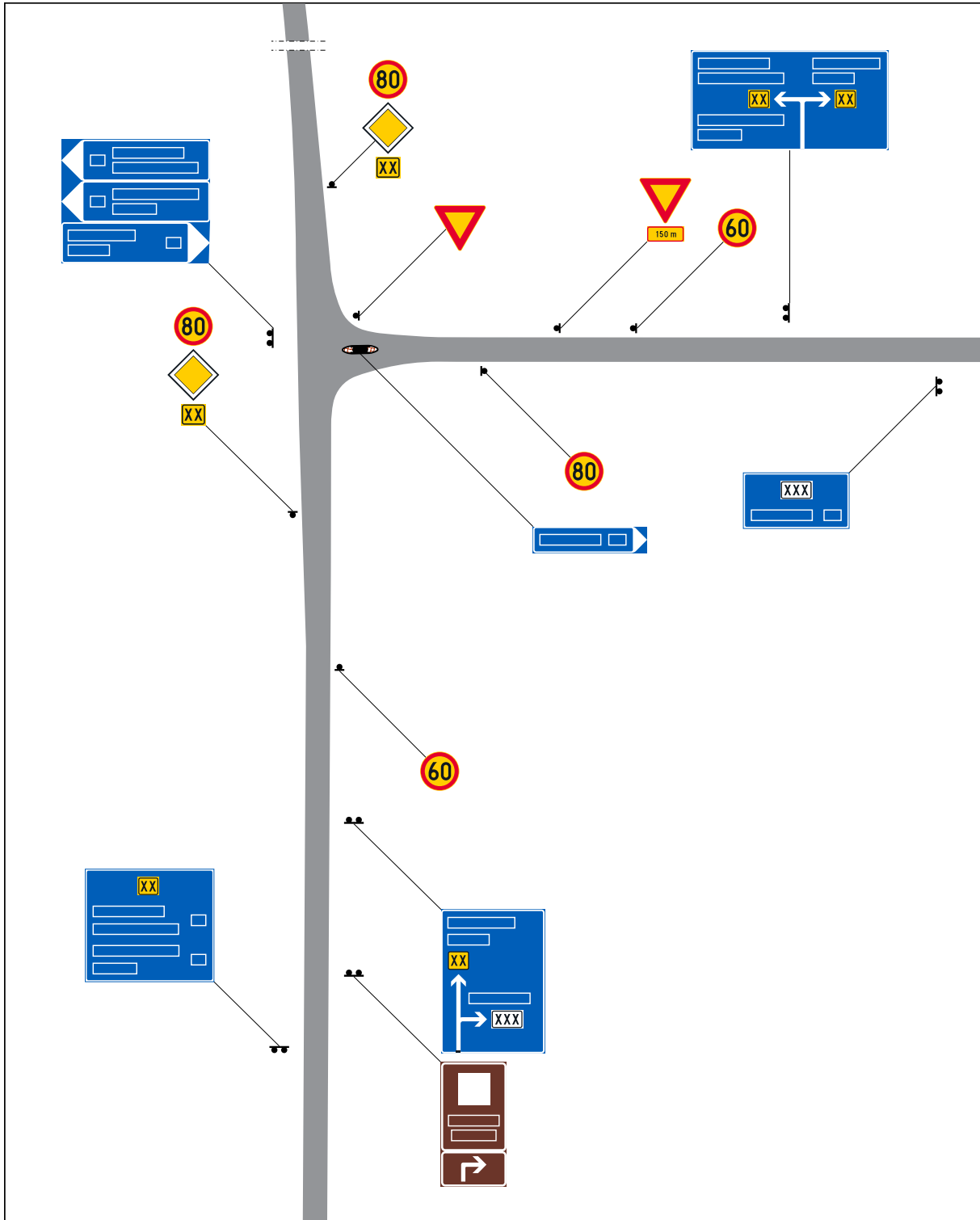
Kuva 6. Esimerkki maanteiden liittymässä olevista liikennemerkeistä.
