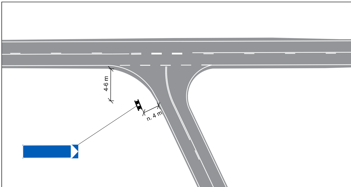
Kuva 4b. Tienviitan sijoittaminen liittymään, kun liikenteenjakajasaareketta ei ole. Viitan sijaintipaikan lumisuus on otettava huomioon jättämällä viitan alle riittävä lumivara. Jos tienviitta joudutaan sijoittamaan liittymän näkemäalueelle, se pyritään sijoittamaan korkeussuunnassa henkilöauton kuljettajan silmäpisteen yläpuolelle (viitan alareunan korkeus tien pinnasta noin 2,0 metriä).
