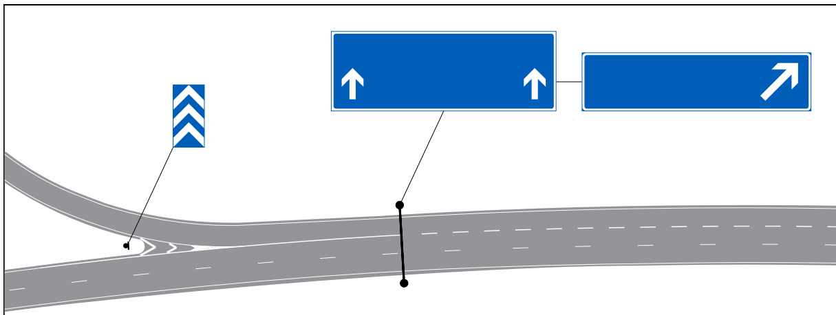
Kuva 121. Merkin F12 (ajokaistan yläpuolinen erkanemisviitta) yhteydessä käytetään erkanemiskohdassa merkkiä I11 (erkanemismerkki).
