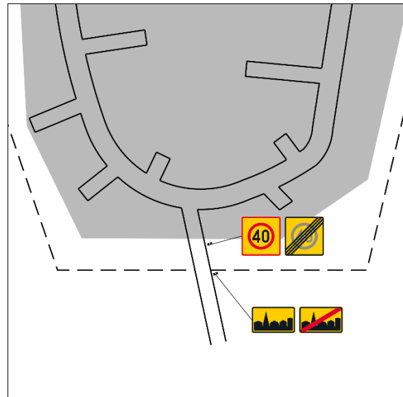
Kuva 105. Merkki E23 (taajama päättyy) ei päättää nopeusrajoitusalueetta. Nopeusrajoitusalue on päätettävä erikseen merkillä C35.
