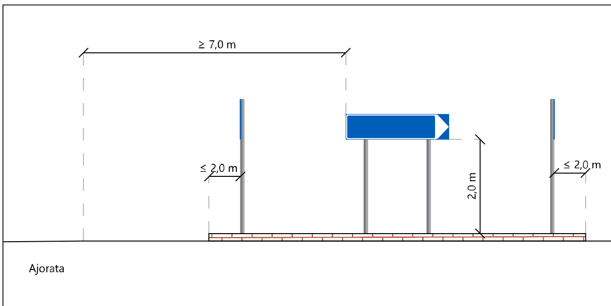
Kuva 4c. Tienviitan sijoittaminen liikenteenjakajasaarekkeeseen. Viitta pyritään sijoittamaan korkeussuunnassa henkilöauton kuljettajan silmäpisteen yläpuolelle (viitan alareunan korkeus tien pinnasta noin 2,0 metriä).
