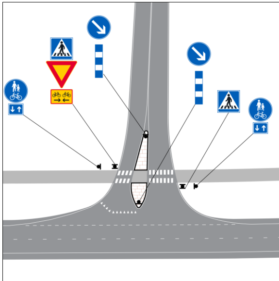
Kuva 70. Yhdistetyn pyörätien ja jalkakäytävän kaksisuuntaisuus osoitetaan aina lisäkilvellä H23.2 (kaksisuuntainen pyörätie) tai H9.1 (vaikutusalue molempiin suuntiin).
