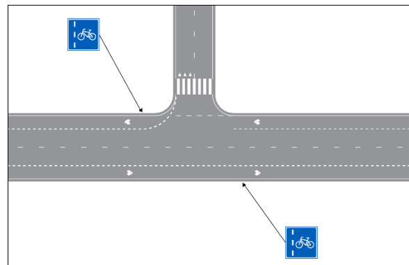
Kuva 93. Merkki E13 (pyöräkaista) toistetaan liittymän molemmiin puolin.
