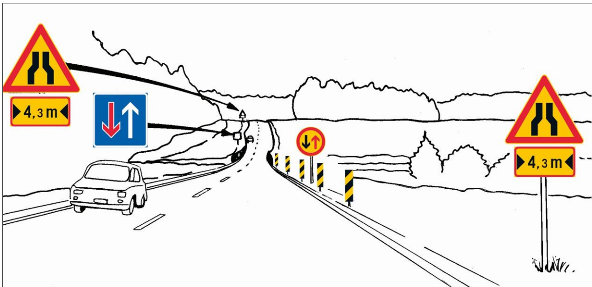
a. Merkin A4 käyttö tilanteessa, jossa kaksikaistainen tie kapenee sillan vuoksi ja vapaa leveys on alle 6,0 m.
