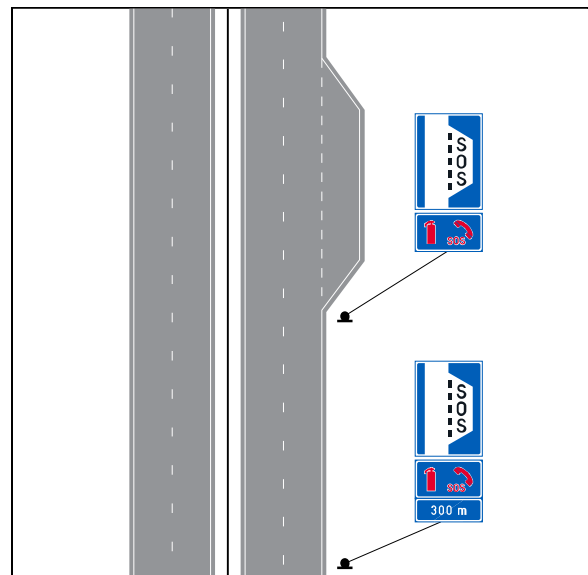
Kuva 101. Merkin E21 (häätäpysäyttämispaiikka) sijoitus.
