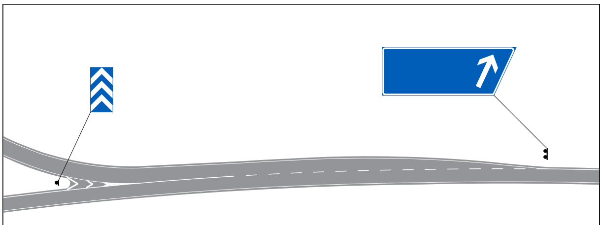
Kuva 124. Erkanemisviitan F14 ja erkanemismerkin I11 käyttö.
