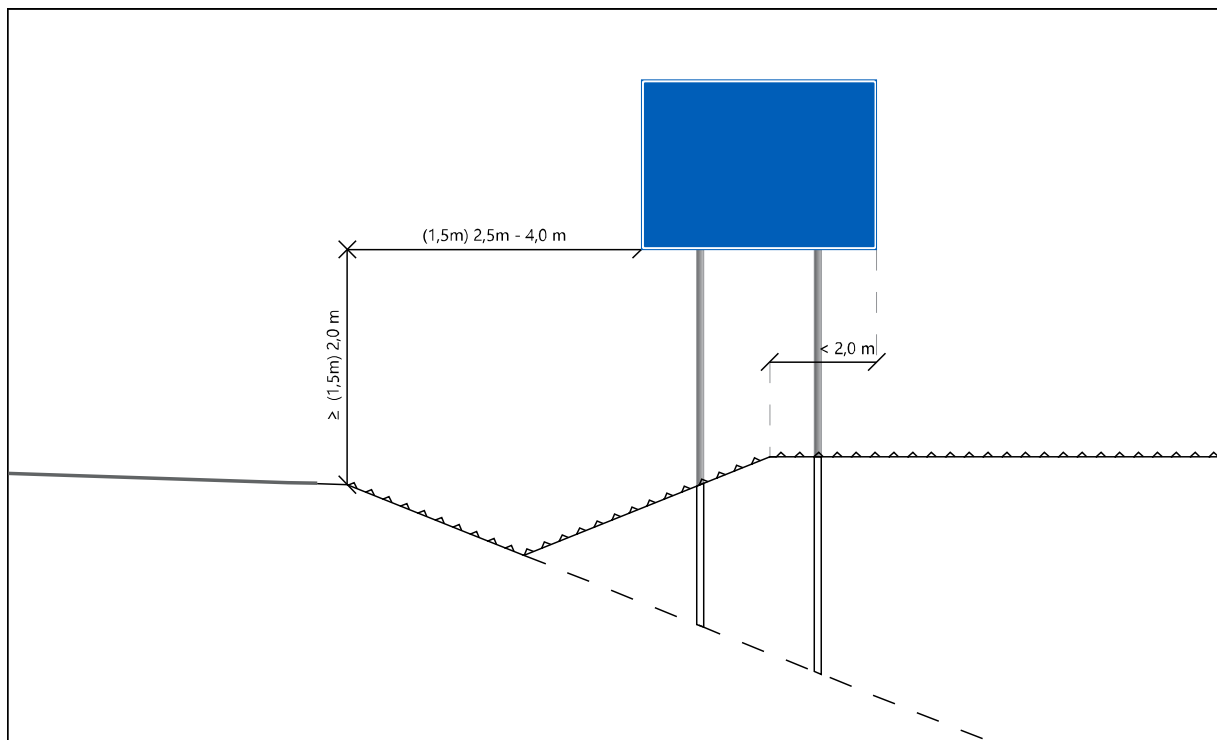
Kuva 3b. Opastusmerkin sijoittaminen muilla maanteilla. Sulkeissa olevia arvoja voidaan käyttää taajamassa ja jos nopeusrajoitus on enintään 50 km/h.
