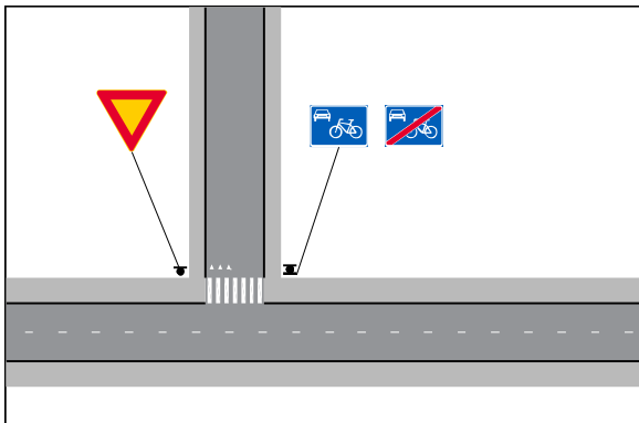
a. Väistämisvelvollisuuden osoittaminen pyöräkadun päättyessä.
