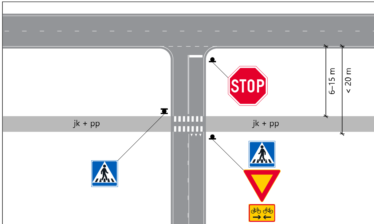
Kuva 34. Pakollisen pysäyttämisen osoittaminen merkillä B6, kun risteävään tiehen kuuluvan jkpp-väylän takaa ei ole riittävä näkemää risteävälle tielle. Muissa tapauksissa merkin B6 sijoittamisessa voidaan soveltaa kuvan 33 esimerkkejä.
