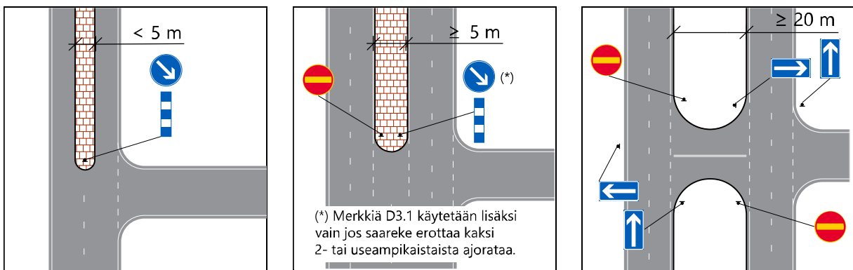
Kuva 68. Merkin D3.1 käyttö erityyppisissä saarekkeissa.
