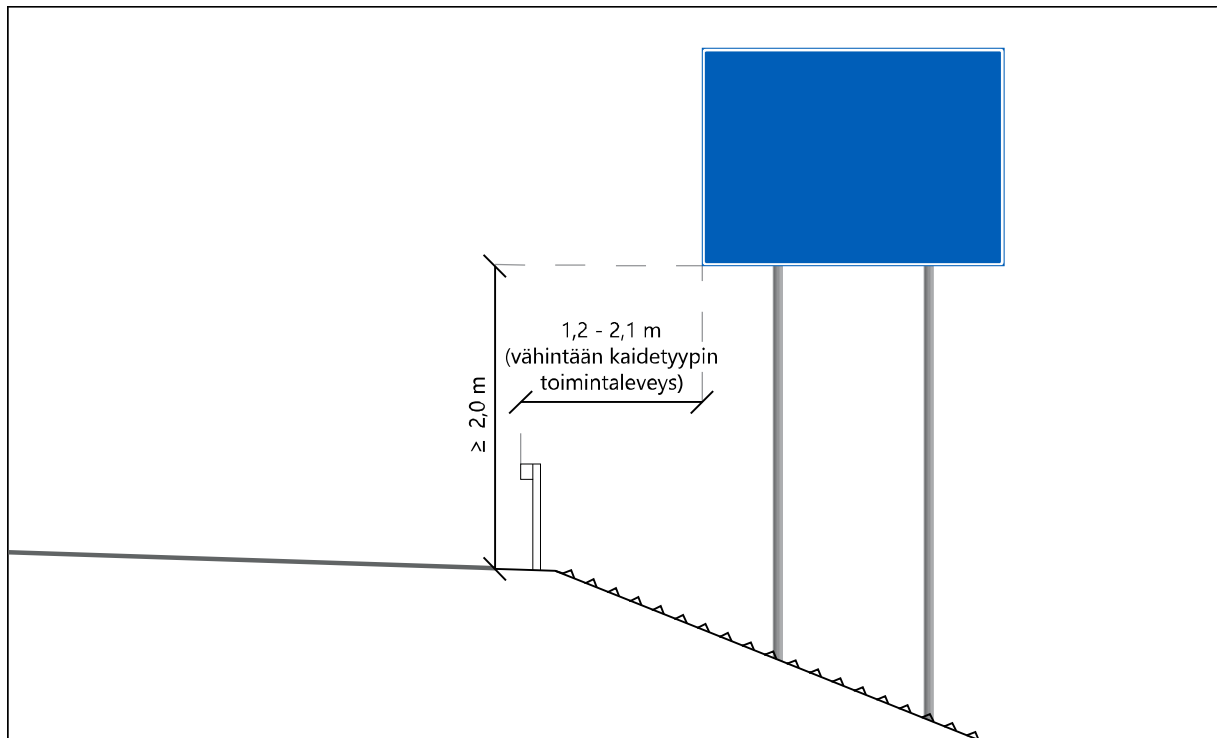
Kuva 3c. Opastusmerkin sijoittaminen kaidteen taakse. Opastusmerkin vähimmäis-etäisyys kaidteen takana määräytyy käytetyn kaidetyypin toimintaleveyden mukaan.
