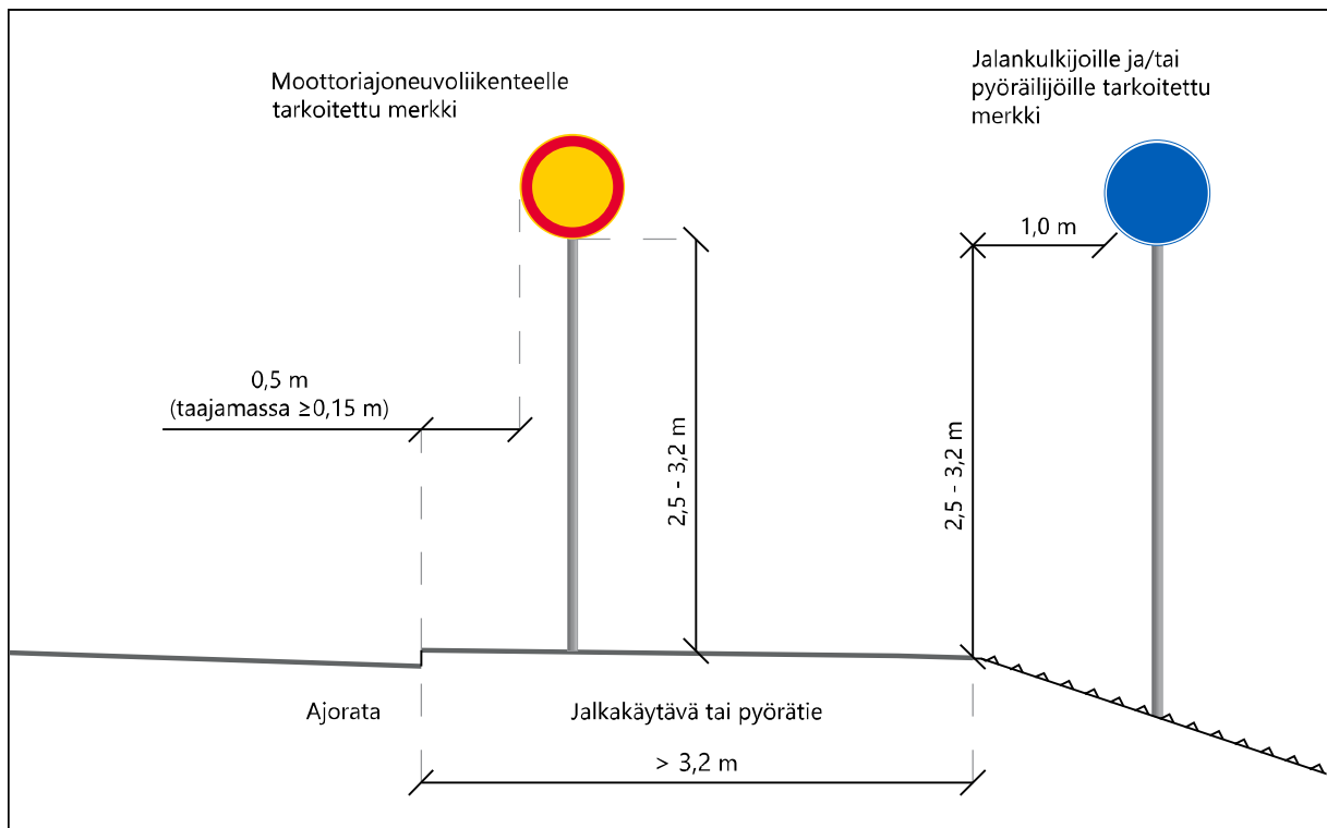
Kuva 1h. Liikennemerkkin sijoittaminen tien poikkileikkaukseen, kun tiehen liittyy yli 3,2 metrin levyinen korotettu pyörätie ja jalkakäytävä, joka ei rajoitu sivuesteeseen.
