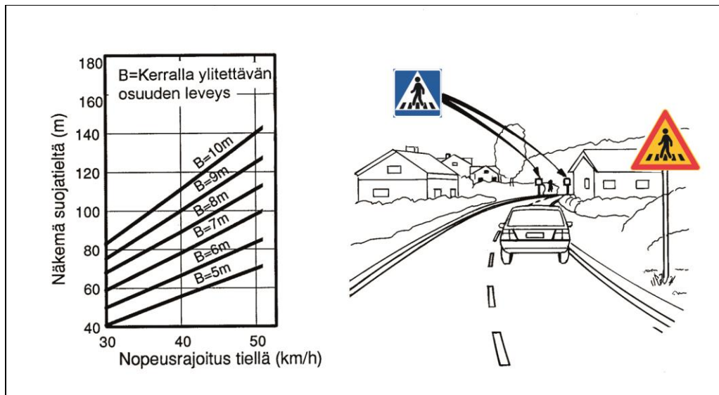
Kuva 19. Suojatien ennakkovaroitusmerkin A15 tarve nomogrammin perusteella.
