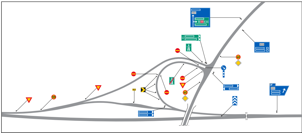
Kuva 8. Esimerkki moottoritien eritasoliittymässä olevista liikennemerkeistä.
