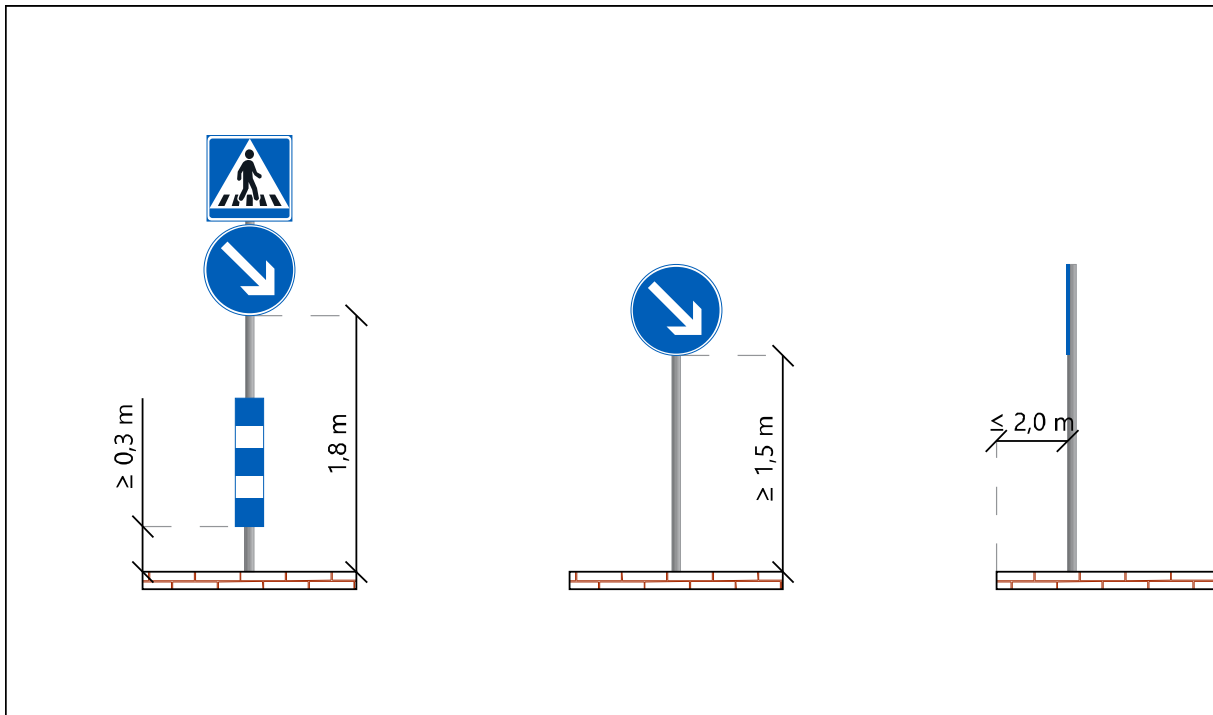
Kuva 2. Merkin D3 (liikenteenjakaaja) sijoittaminen saarekkeeseen. Merkin I10.1 (liikennemerkkipylvään tehostamismerkki) korkeusasema liikennesaarekkeen tai tien pinnasta on vähintään 0,3 m. Yksittäisen merkin D3 alareunan korkeus on yleensä vähintään 1,5 m, mutta voi poikkeuksellisesti olla 0,4 m (ei kuitenkaan maanteilla).
