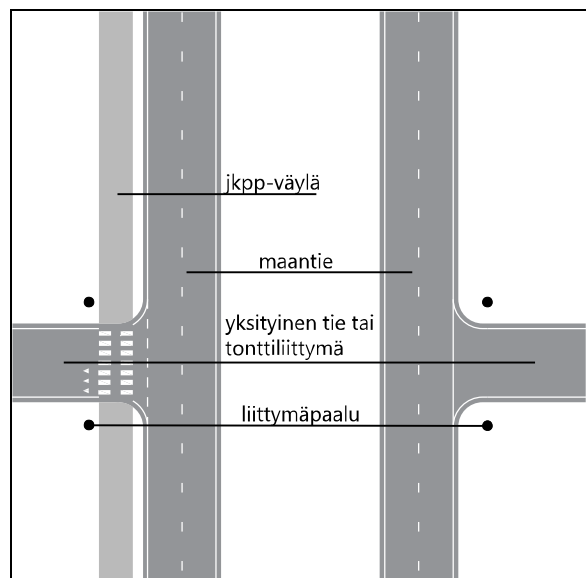
Kuva 171. Liittymäpaalun sijoitus.
