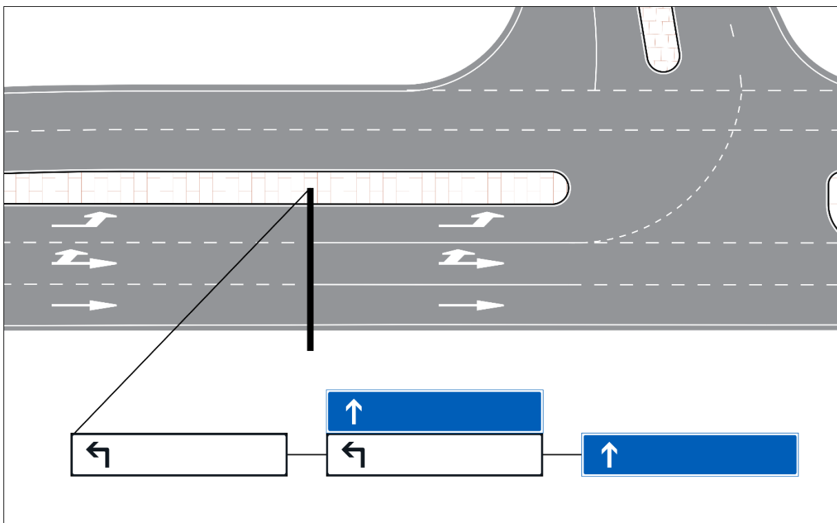
Kuva 64. Ajokaistan yläpuolisten viittojen yhteydessä tieliikennelain yleisistä säännöksistä poikkeava ryhmittäminen osoitetaan ajokaistanuolilla. Tällöin ei käytetä samanaikaisesti merkkejä D1.3–D1.9.
