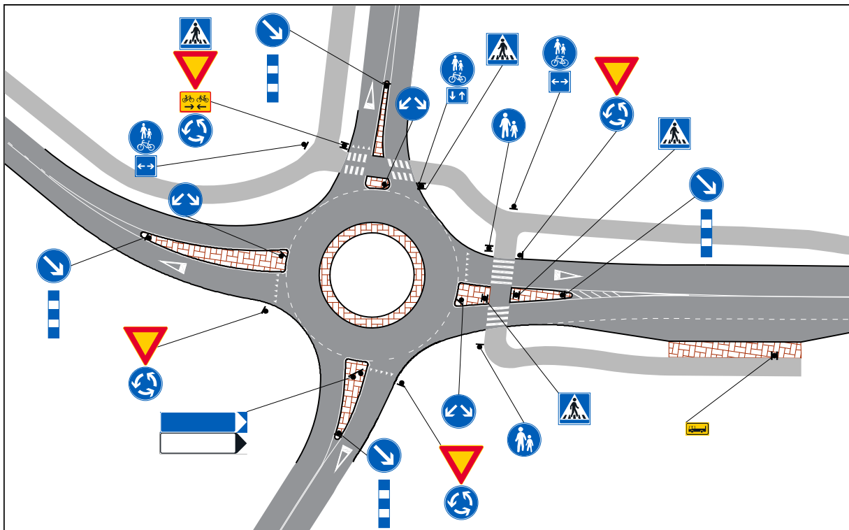
Kuva 5b. Esimerkki liikenneympyrässä käytettävistä liikennemerkkeistä.
