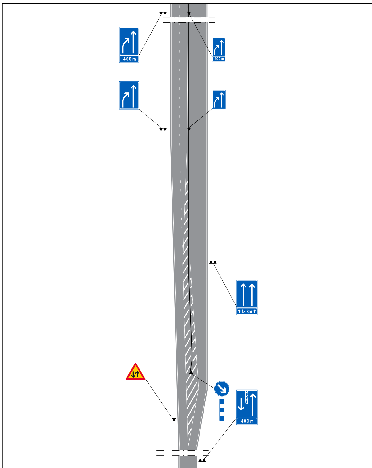
Kuva 120. 2+2 -ajokaistaisen ohituskaistan merkintäperiaate.
